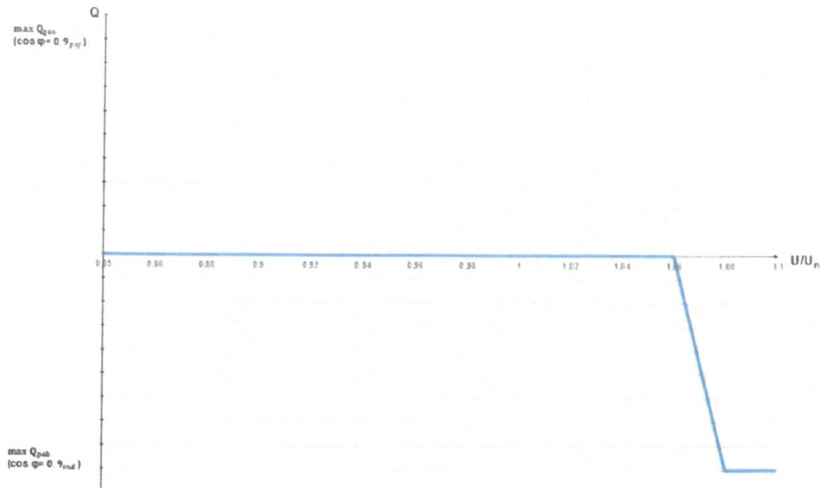
Rys.4. Charakterystyka sterowania mocą bierną w funkcji napięcia dla mikroinstalacji podłączonych jednofazowo, wymagana przez OSDnn.
