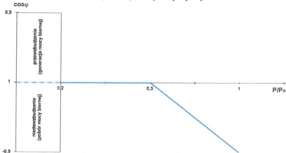
Rys.5. Charakterystyka sterowania współczynnikiem mocy \cos \varphi w funkcji generowanej mocy czynnej wymagana przez OSDnn.
