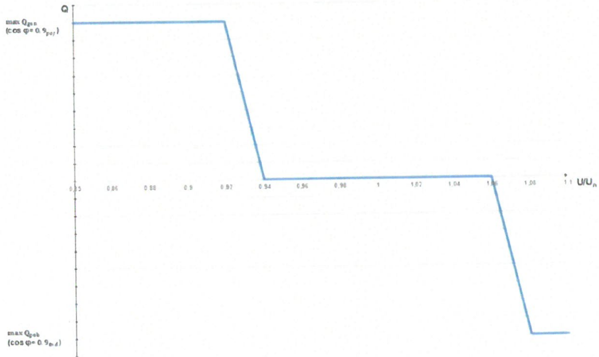
Rys.3. Charakterystyka sterowania mocą bierną w funkcji napięcia wymagana przez OSDnn.
