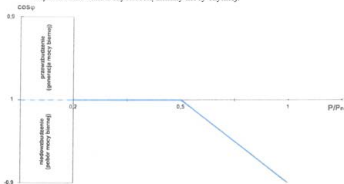
Rys.5. Charakterystyka sterowania współczynnikiem mocy \cos \varphi w funkcji generowanej mocy czynnej wymagana przez OSDnn.
